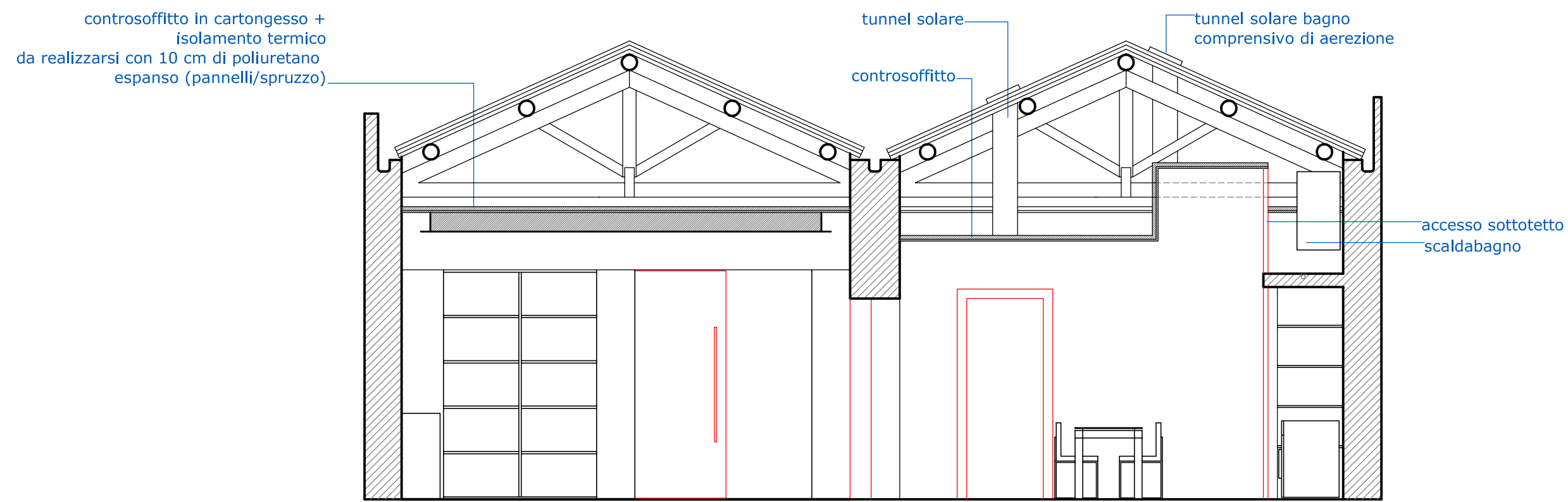
Sezione X-X'
